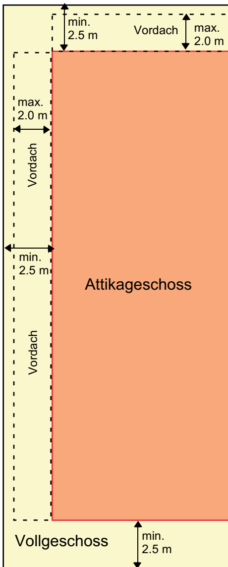
Grundriss
