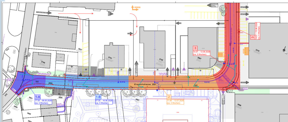
Abbildung 1: Etappen 1A, 1B, 2 und 3
